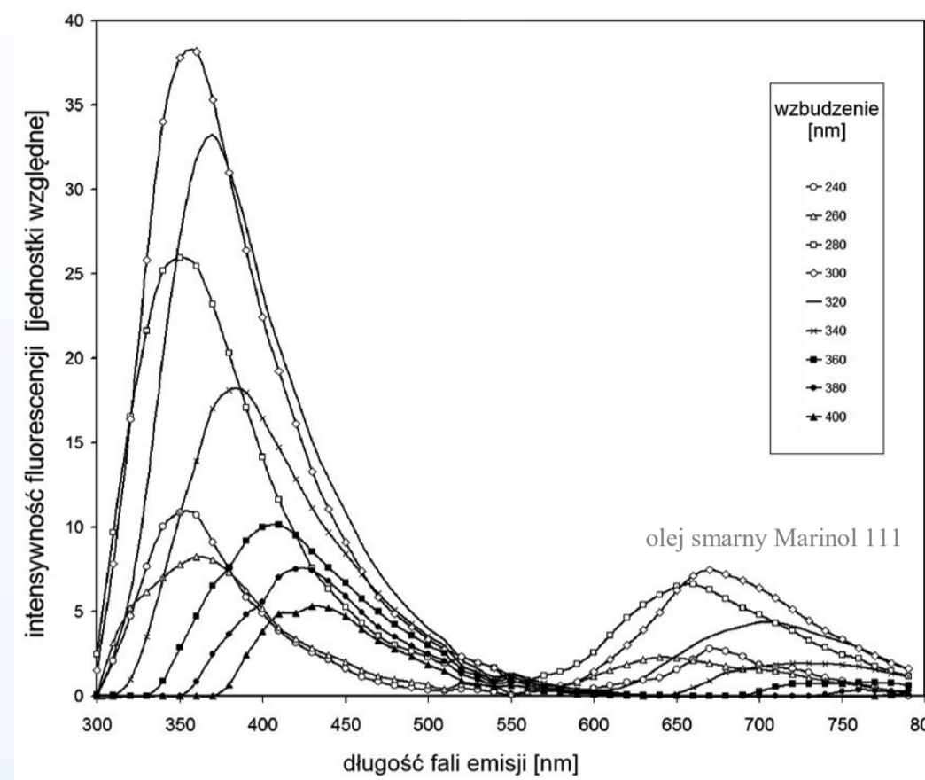
Widmo wzbudzenia
