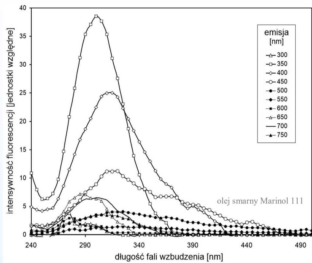
Widmo emisji
