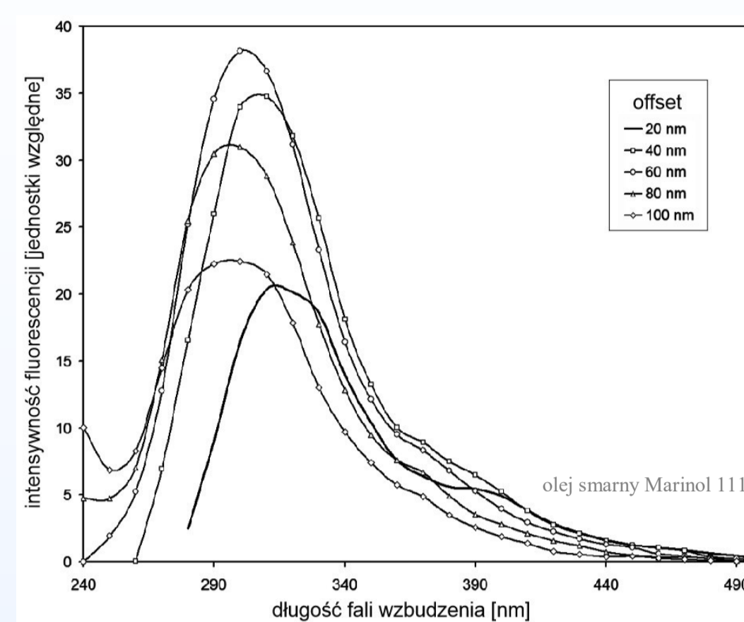
Widmo synchroniczne
