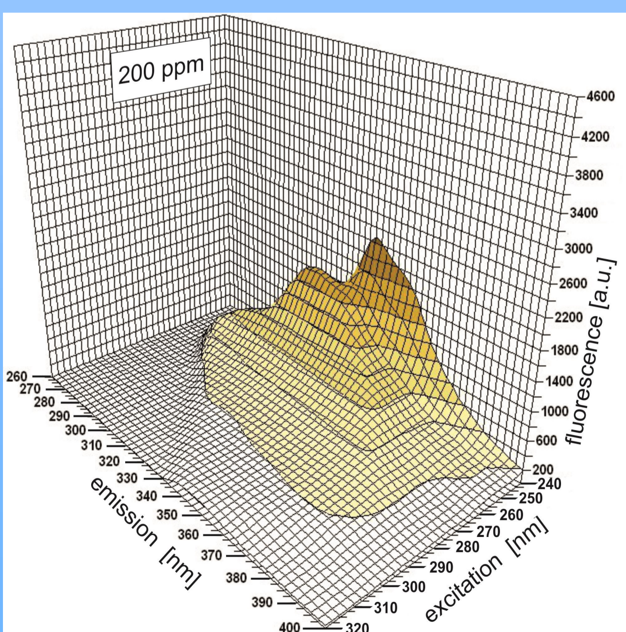
Widma zupełne fluorescencji wody skontaktowanej z olejem smarnym
