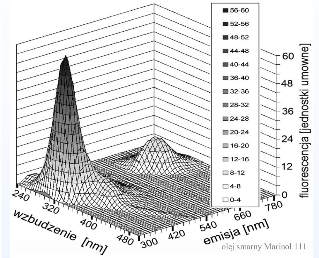
Widmo zupełne
